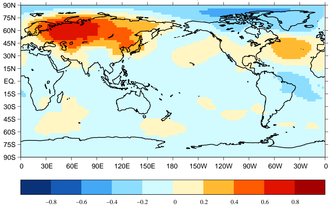
EOF3 NH SLP anomalies, 1948–Feb2005
