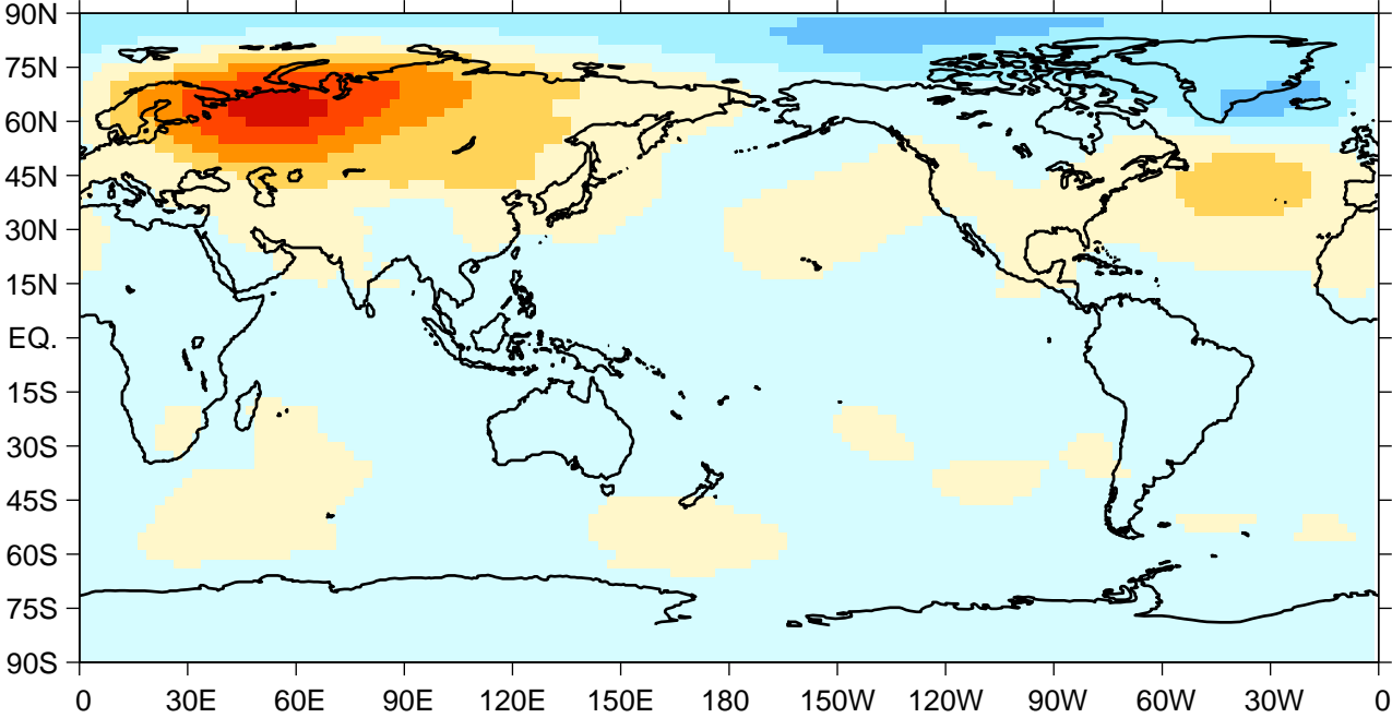
EOF3 NH SLP anomalies (mb) 1948–Feb2005
